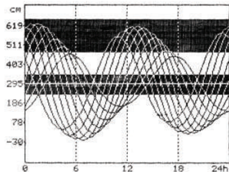
CHATHAM L = 51° 24' N G = 000° 33' E U.T. Etude de l'onde du 22 / 04 / 1838 au 01 / 05 / 1838
