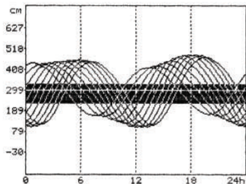
FALMOUTH L = 50° 09' N G = 005° 03' W U.T. Etude de l'onde du 22 / 06 / 1885 au 01 / 07 / 1885
